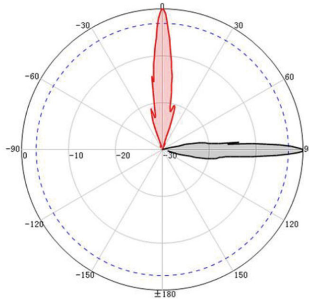
H-Pol
