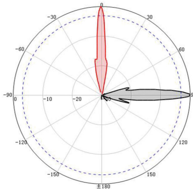
V-Pol
